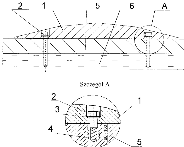
Rys. 4. Przykład umocnienia progu do nawierzchni jezdni
